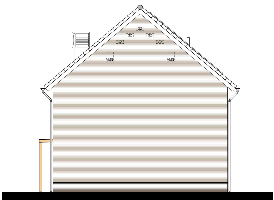
RECHTER ZIJGEVEL
