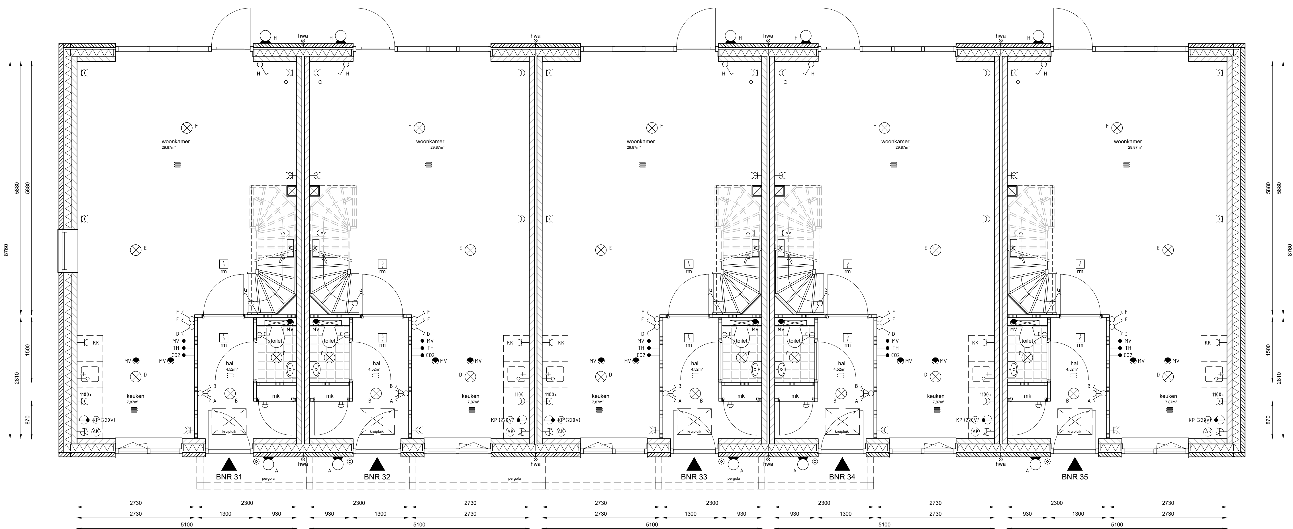
BEGANE GROND
