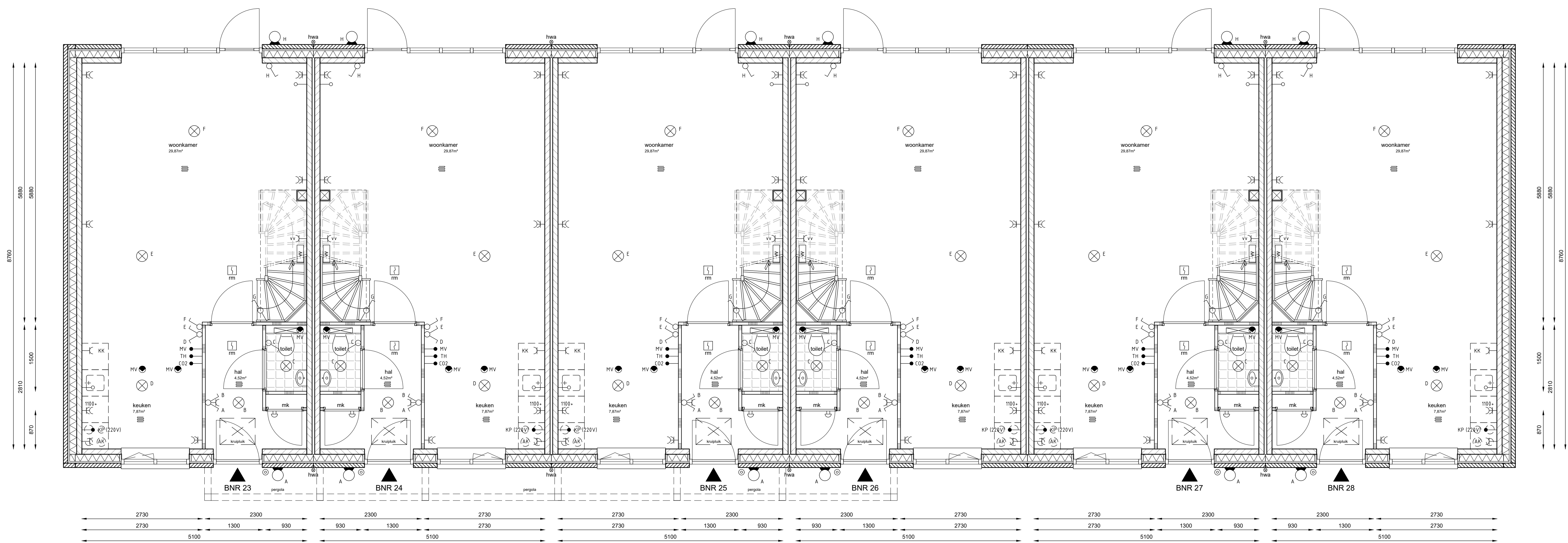
BEGANE GROND
