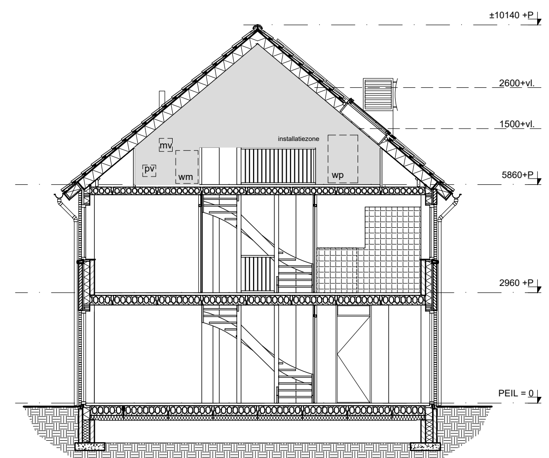
DOORSNEDE
