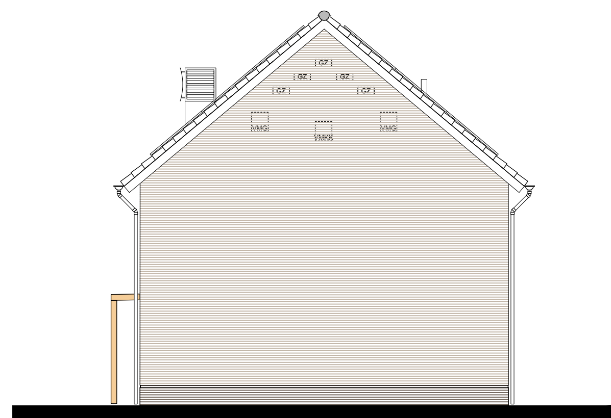
RECHTER ZIJGEVEL
