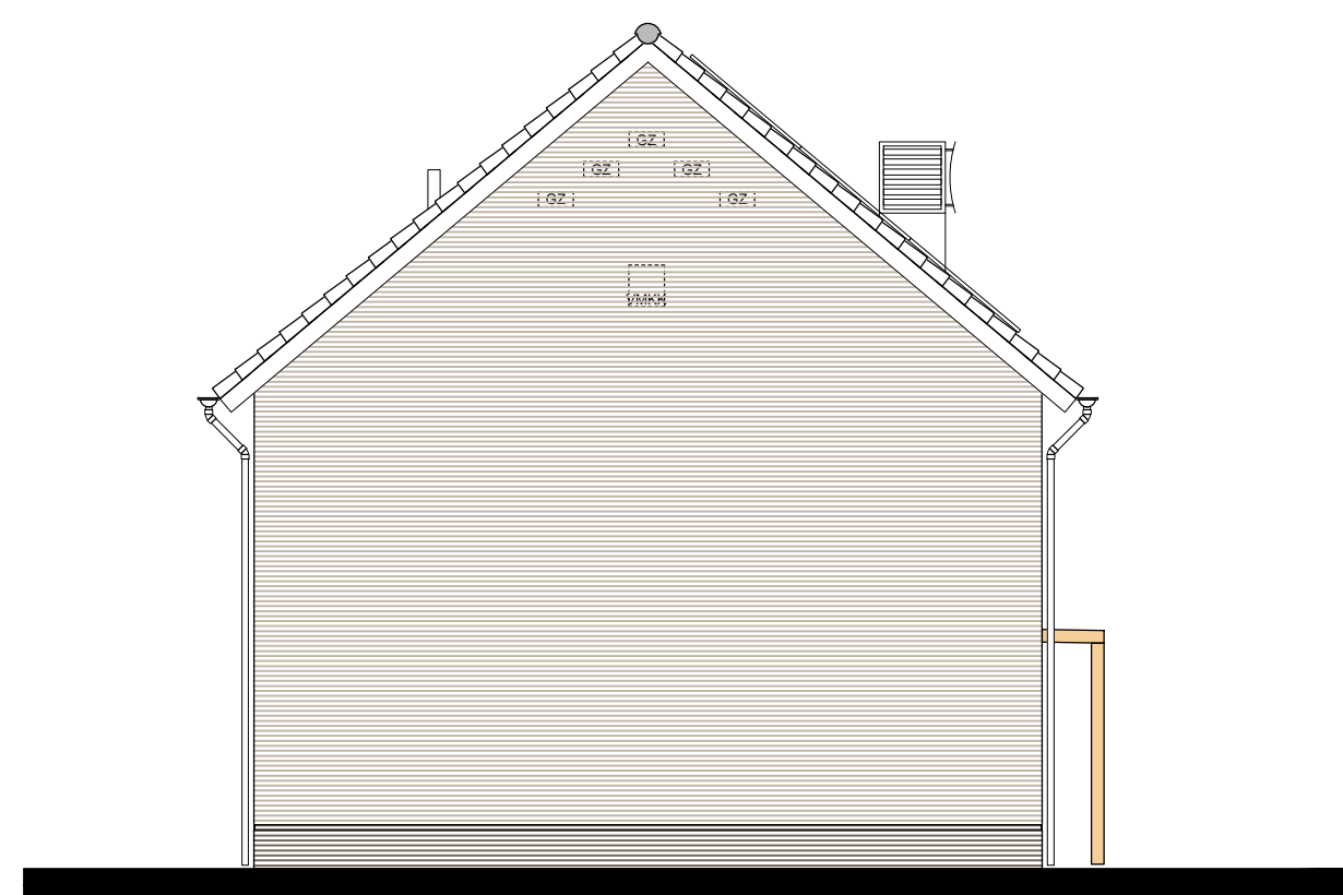
LINKER ZIJGEVEL
