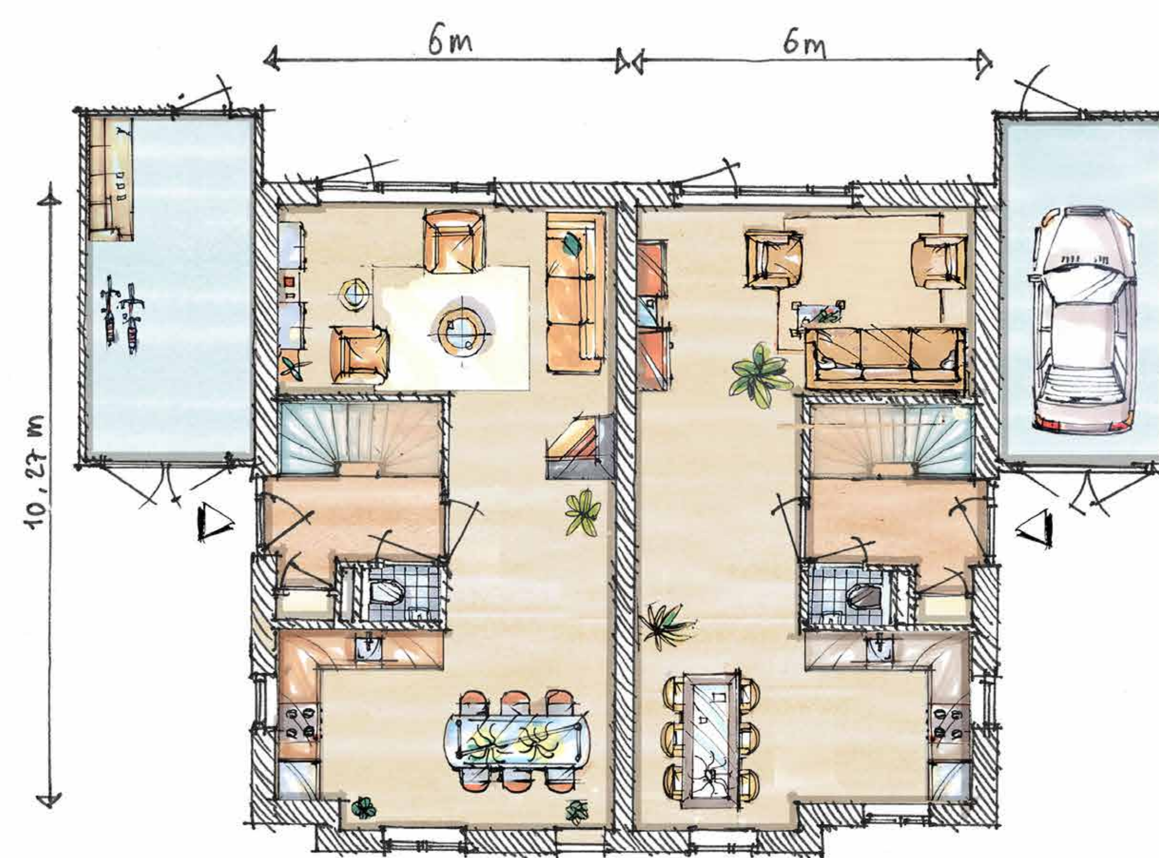
Begane Grond
